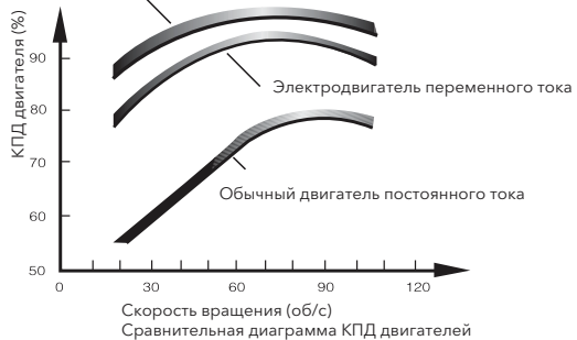
Синхронный электродвигатель с редкоземельным постоянным магнитом
