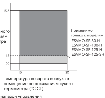
Работа в режиме обогрева
