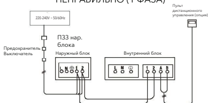
НЕПРАВИЛЬНО (1 ФАЗА)
