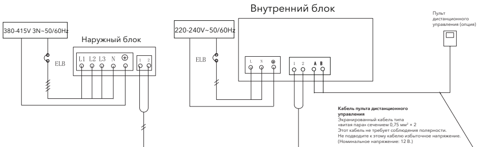
Соединения проводов внутреннего и наружного блоков (3 ФАЗЫ)
