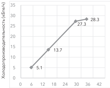
Общая производительность подключенных внутренних блоков (кВт/ч)
