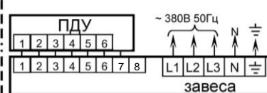
Схема подключения тепловых завес к трехфазной сети и пульта
