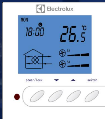
Пульт управления ERC-20
