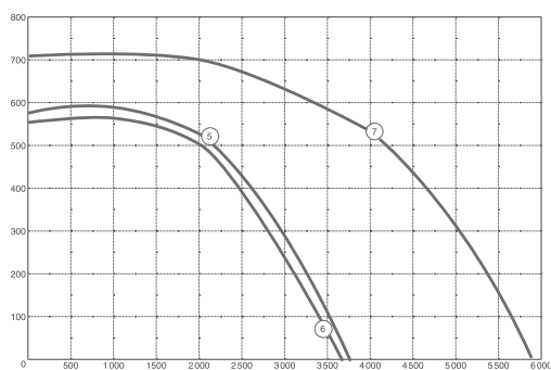
Аэродинамические характеристики установок
