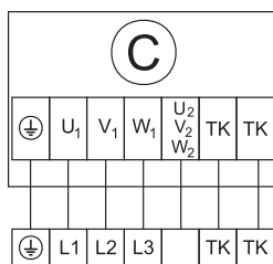
Схема №2 (3-400 В)
