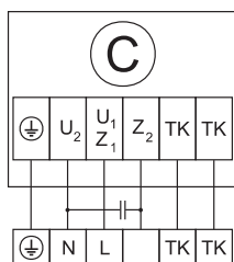
Схема №1 (1-230 В)
